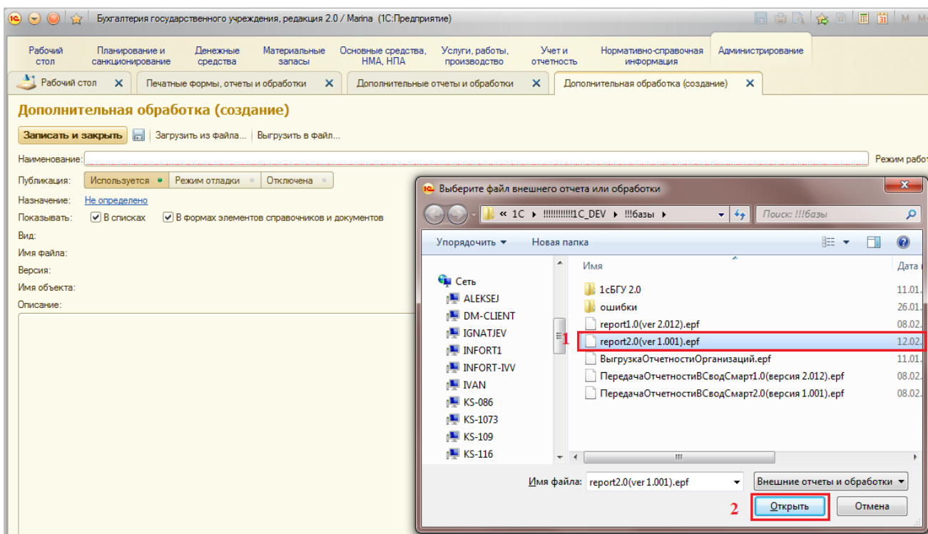
Рисунок 22 Добавление внешней обработки.
